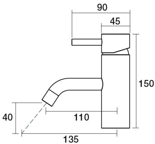
Lugano Hob Basin Mini Mixer A22.013.1.01 - Chrome
