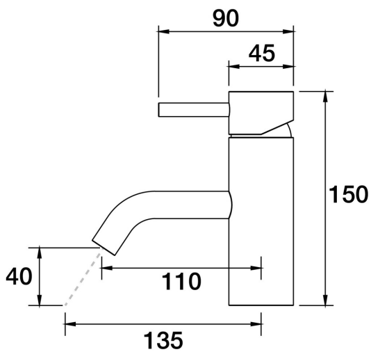
Lugano Hob Basin Mini Mixer A22.013.1.48 - Copper
