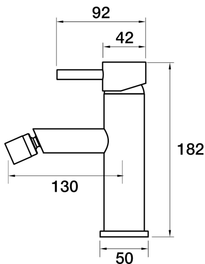
Lugano Bidet Mixer A22.061.1.11 - 23k Gold
