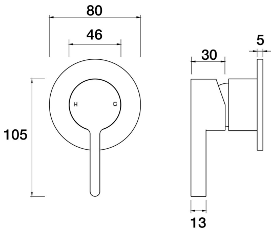
Fuze Wall Mixer Shower A25.031.1.01 - Chrome
