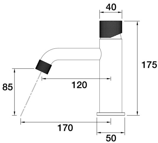
IDK Hob Basin Mixer A38.011.1.01 - Chrome
