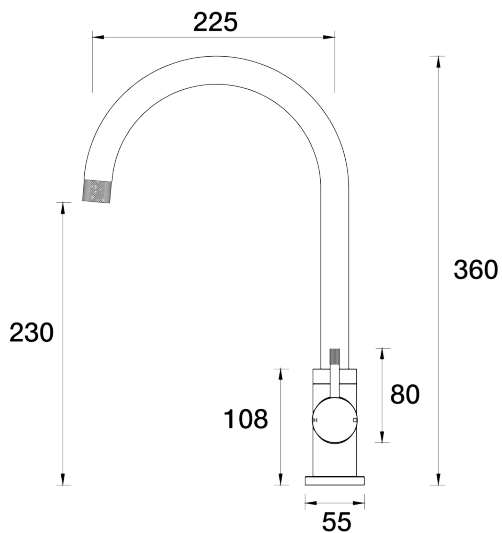
Elm Sink Gooseneck Mixer A40.026.1.01 - Chrome
