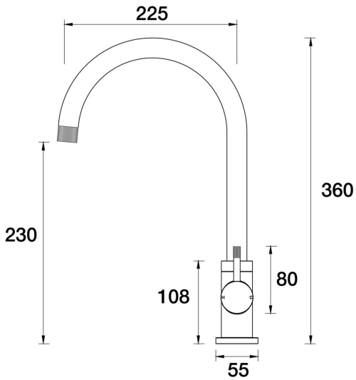
Elm Sink Gooseneck Mixer A40.026.1.01 - Chrome
