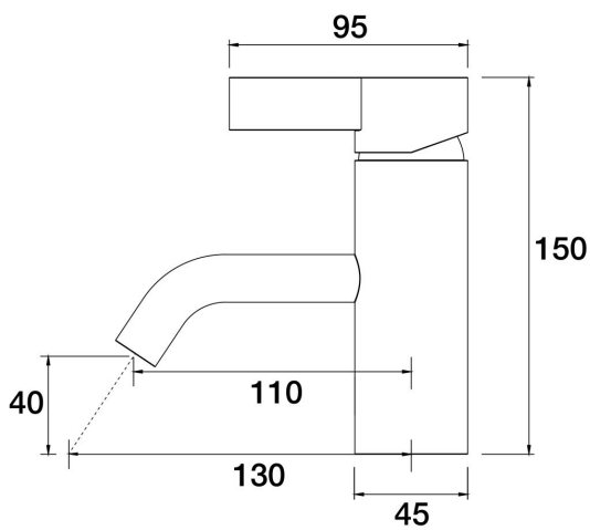
ARI Hob Basin Mini A43.013.1.01 - Chrome
