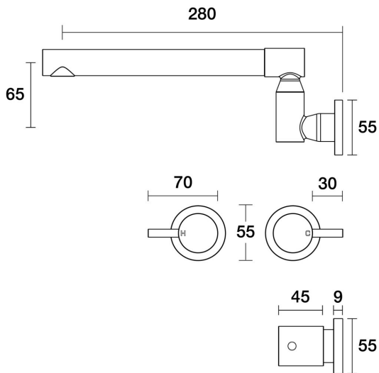
Lugano Sink Set XL Wall Swivel B22.054.1.01 - Chrome
