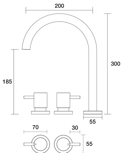
Lugano Spa Set Hob Swivel B22.061.1.48 - Copper
