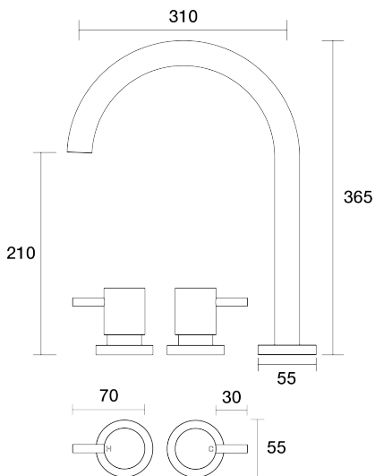
Lugano Spa Set XL Hob Swivel B22.063.1.01 - Chrome
