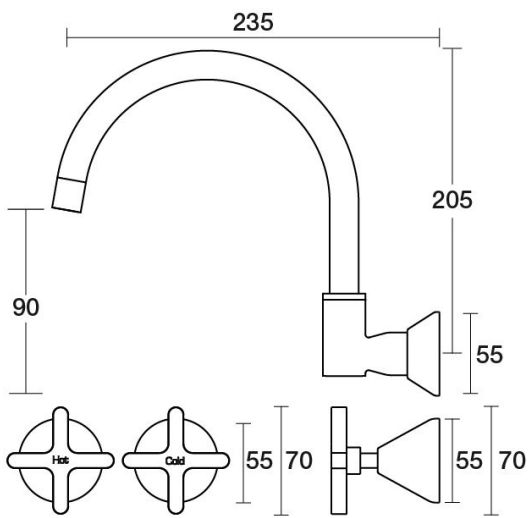
Forme Sink Set Wall Swivel B27.052.1.01 - Chrome
