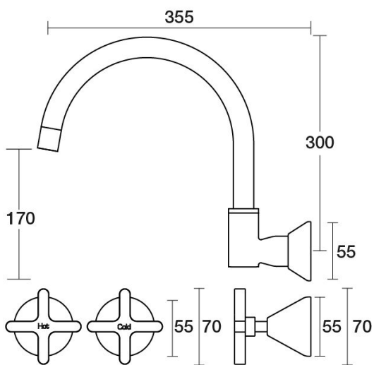
Forme Sink Set XL Wall Swivel B27.054.1.01 - Chrome
