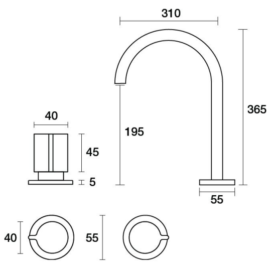
Q Spa Set XL Hob Swivel B36.063.1.01 - Chrome
