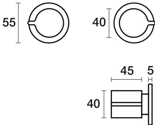
Q Top Assemblies Wall Pair B36.082.1.01 - Chrome
