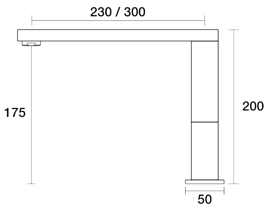
Burj Spa Hob Swivel Outlet D20.042.1.01 - Chrome
