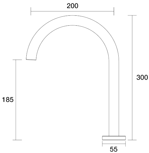
Lugano Sink Hob Swivel Outlet D22.032.1.01 - Chrome
