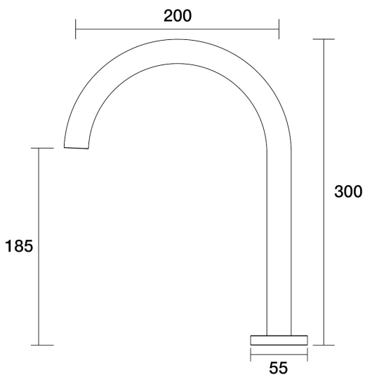
Lugano Sink Hob Swivel Outlet D22.032.1.57 - Matt Nickel
