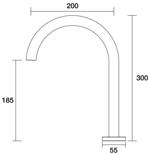
Lugano Spa Hob Swivel Outlet D22.042.1.01 - Chrome
