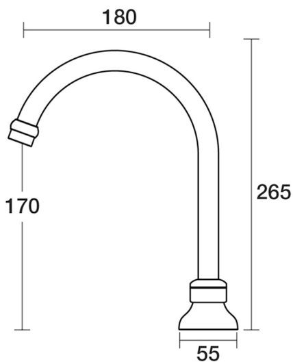
Bell Sink Hob Swivel Outlet D32.032.1.01 - Chrome
