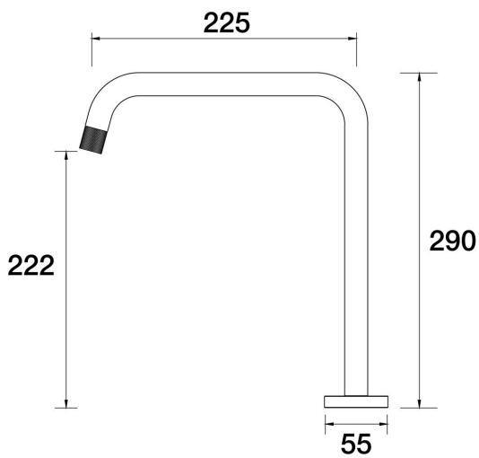
Elm Spa Hob Swivel Outlet D40.042.1.01 - Chrome
