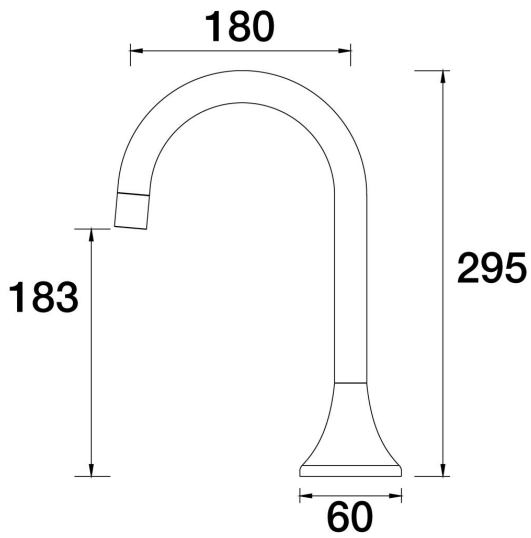
ARI Sink Hob Swivel Outlet D43.032.1.01 - Chrome
