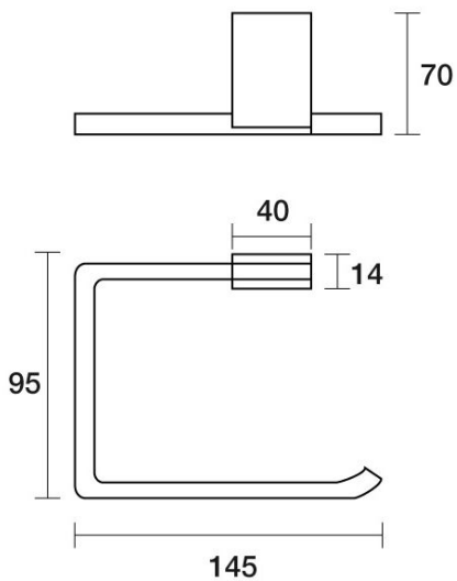
Burj - Online Exclusive Toilet Roll Holder E20.051.1.01 - Chrome
