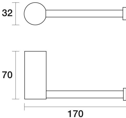
Lugano Toilet Roll Holder E22.051.1.01 - Chrome
