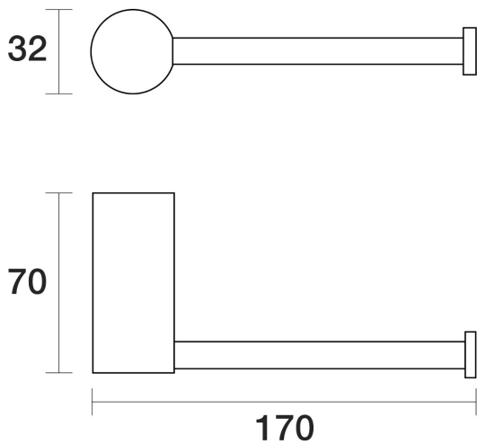
Lugano Toilet Roll Holder E22.051.1.47 - Luminick
