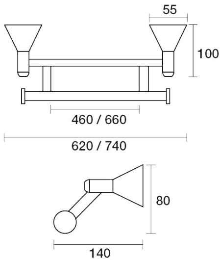
Forme Towel Rail Double 660mm E27.072.1.01 - Chrome
