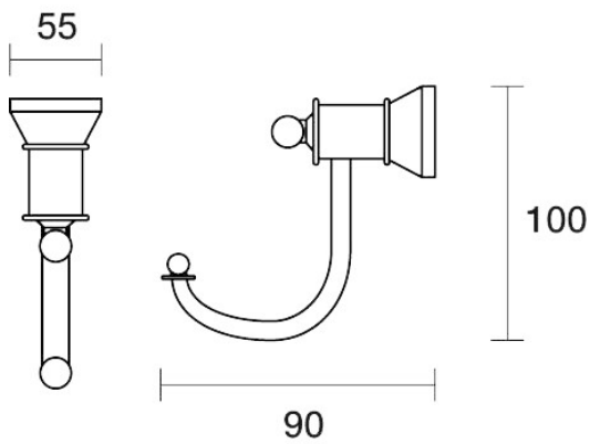
Tudor Robe Hook Holder E31.061.1.01 - Chrome
