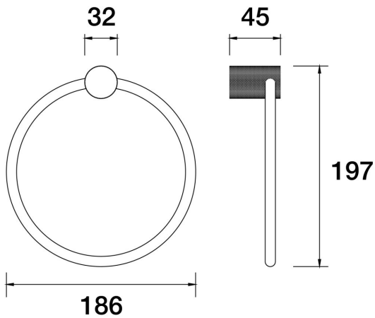
IDK Towel Ring Holder E38.031.1.01 - Chrome
