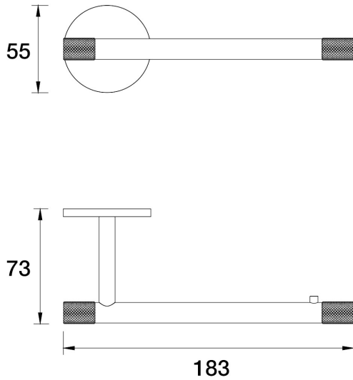
Opus Toilet Roll Holder E45.051.1.32 - Midnight Black
