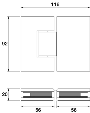
Universal Shower Hinge - 180° L11.011.1.01 - Chrome
